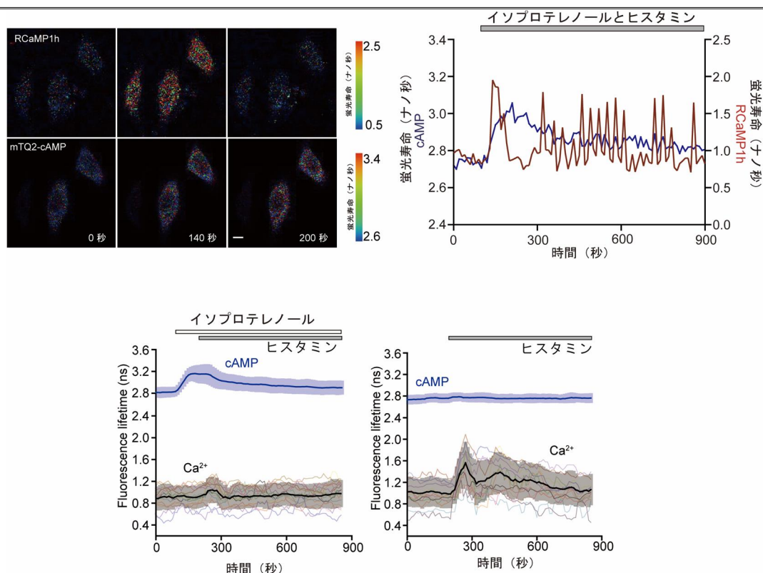
図3 蛍光寿命バイオセンサーを用いた cAMP と \text{Ca}^{2+} の2色イメージング
