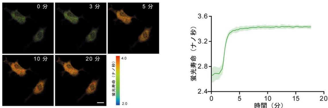
図 2 細胞内 cAMP 可視化する蛍光寿命センサー「qmTQ2-cAMP」の開発
