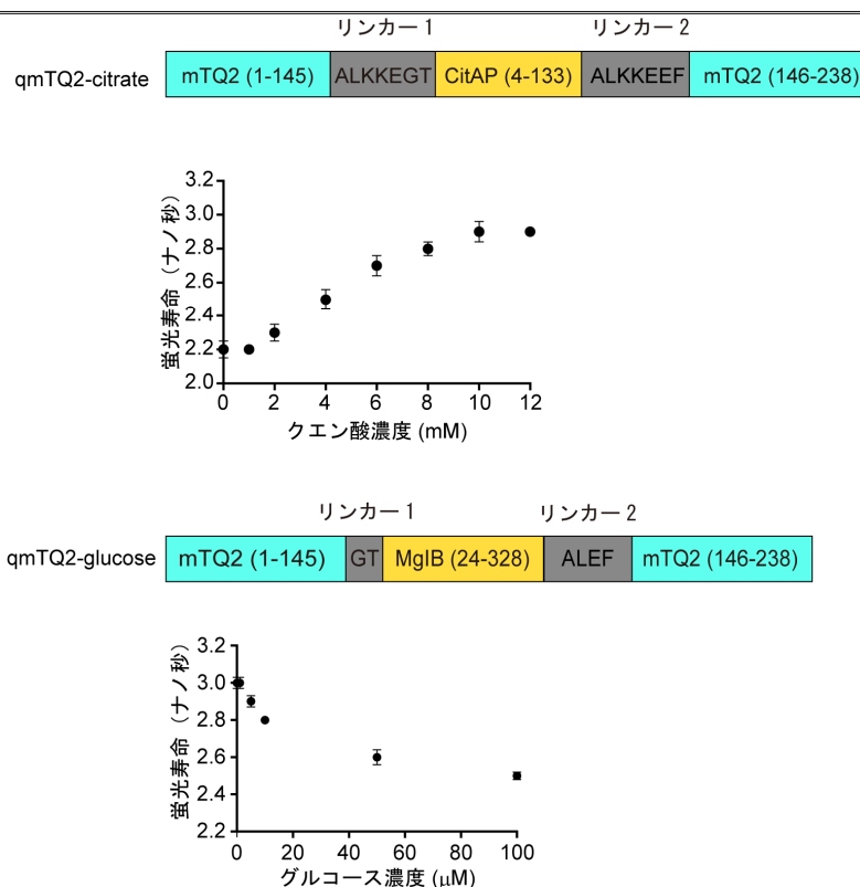
図 4 クエン酸とグルコースに対する蛍光寿命センサーの開発
