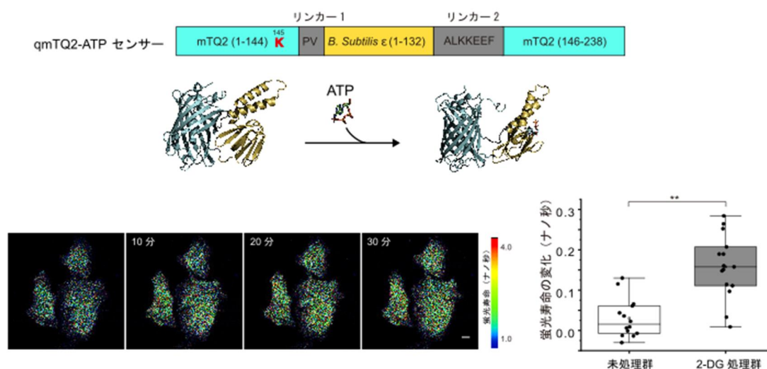
図 1 細胞内エネルギー代謝評価のための ATP 蛍光寿命センサーの開発
